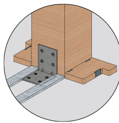
poteau fixé au sol par équerres métalliques* contre un cloison en plaques de plâtre
